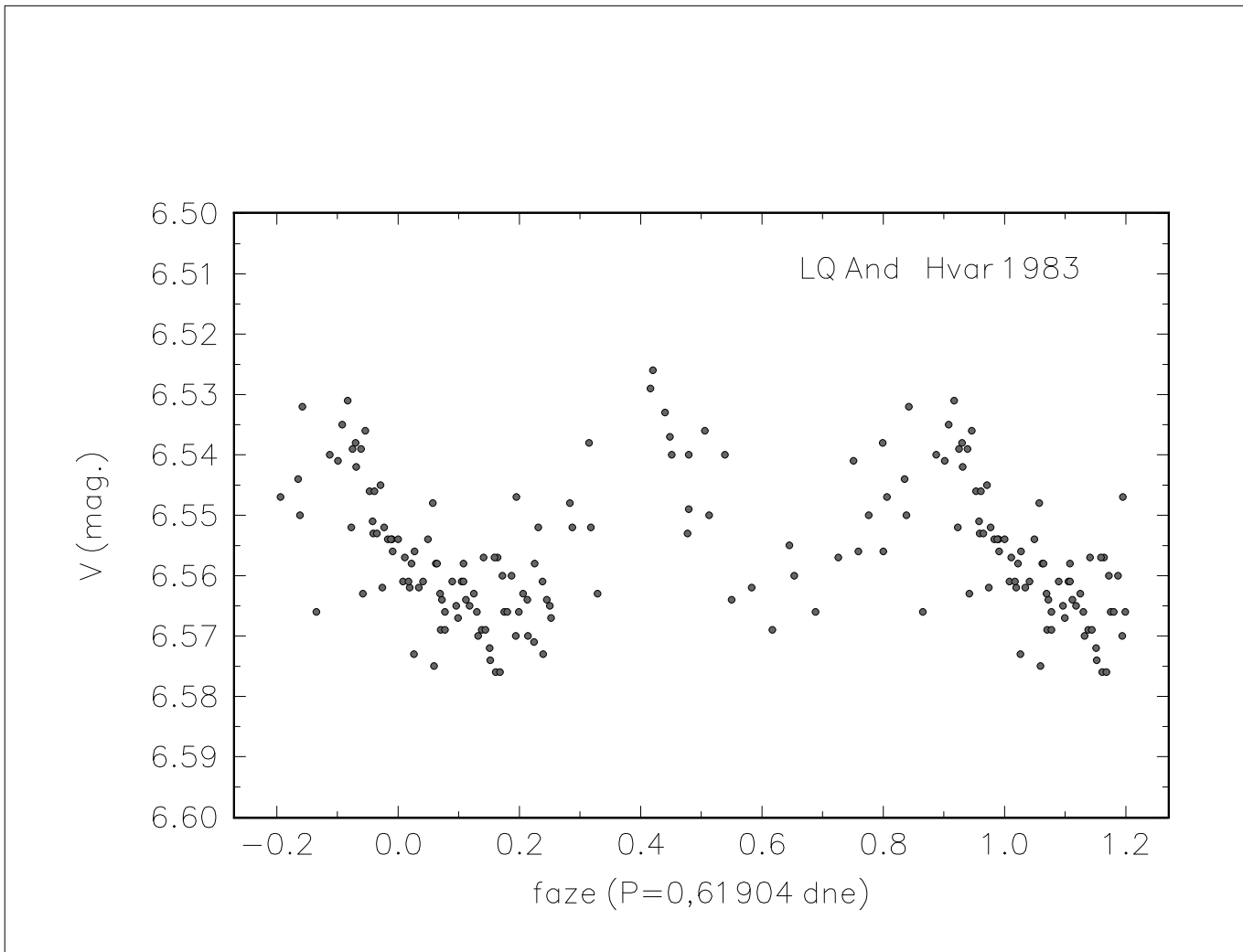
Obrázek 7: Světelná křivka LQ And pro data znázorněná na obr. 4 a pro nejlepší nalezenou periodu 0,61904 dne.
